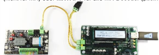
ein bedrahteter Decoder zum SW-Update, Sound-Laden, Testen an MSTAPK ; Verbindung zu MXULFA über „Schiene“, Software und Sound-Projekte vom USB-Stick.
