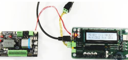
ein „Next18“-Decoder zum SW-Update und Sound-Laden an MSTAPK ; Verbindung zu MXULFA über „SUSI“-Kabel. KEIN Kabel „Schiene“! Software und Sound-Projekte vom Computer (Programme ZSP oder ZCS) über USB-Kabel.
